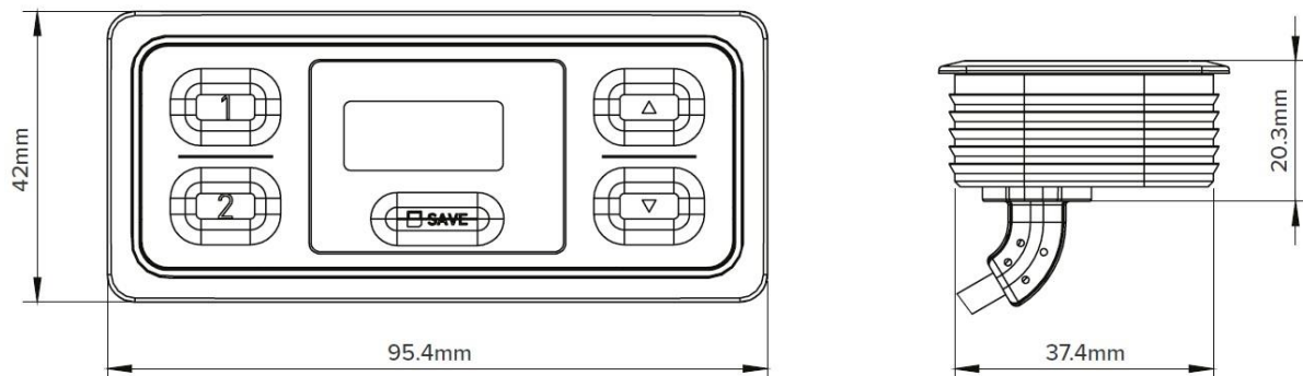
Fig. 2: Productafmetingen TOUCHinlay-2M2-KM
